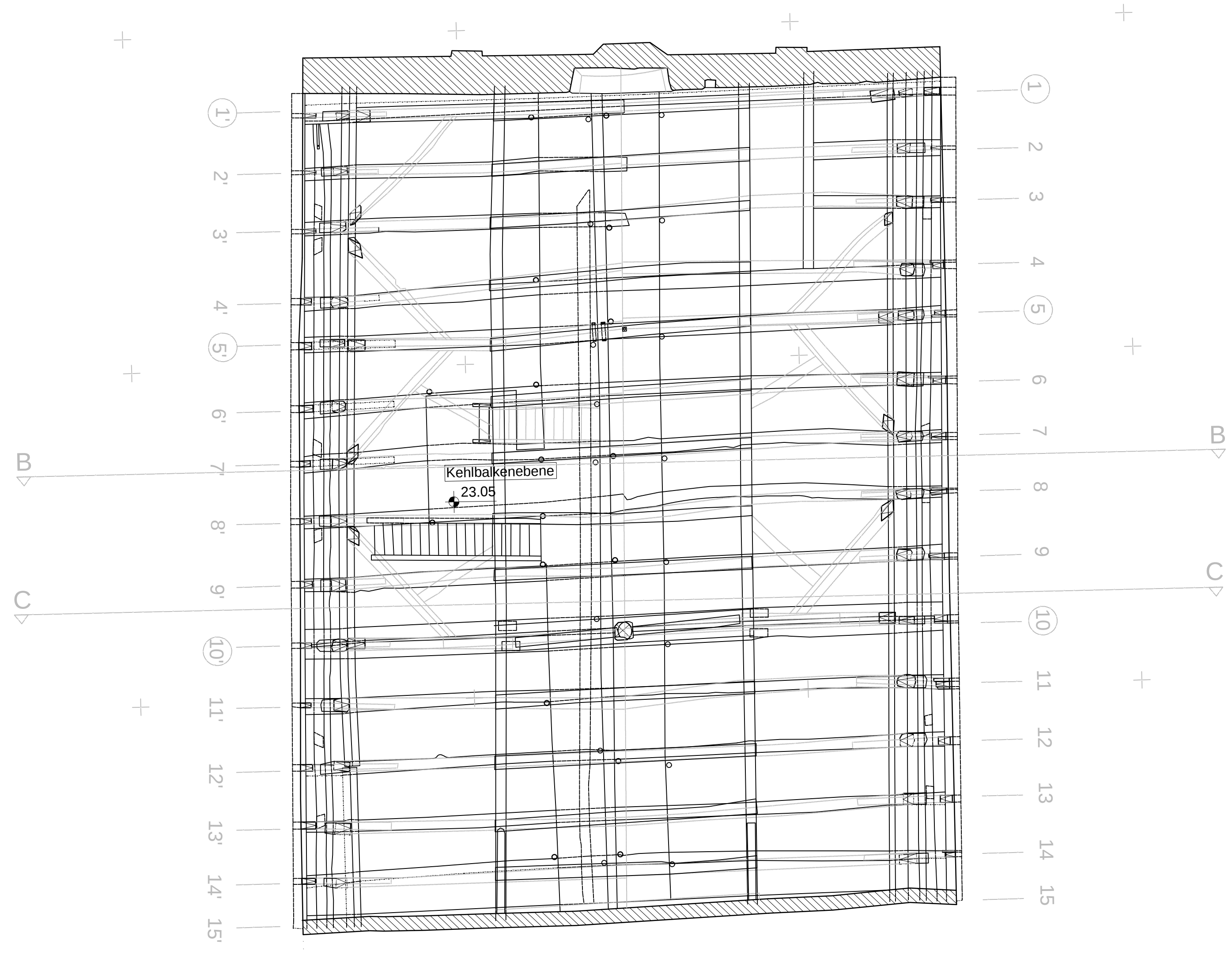
TREPPENHAUS GRUNDRISS KEHLBALKENEbene KBE M 1:50
