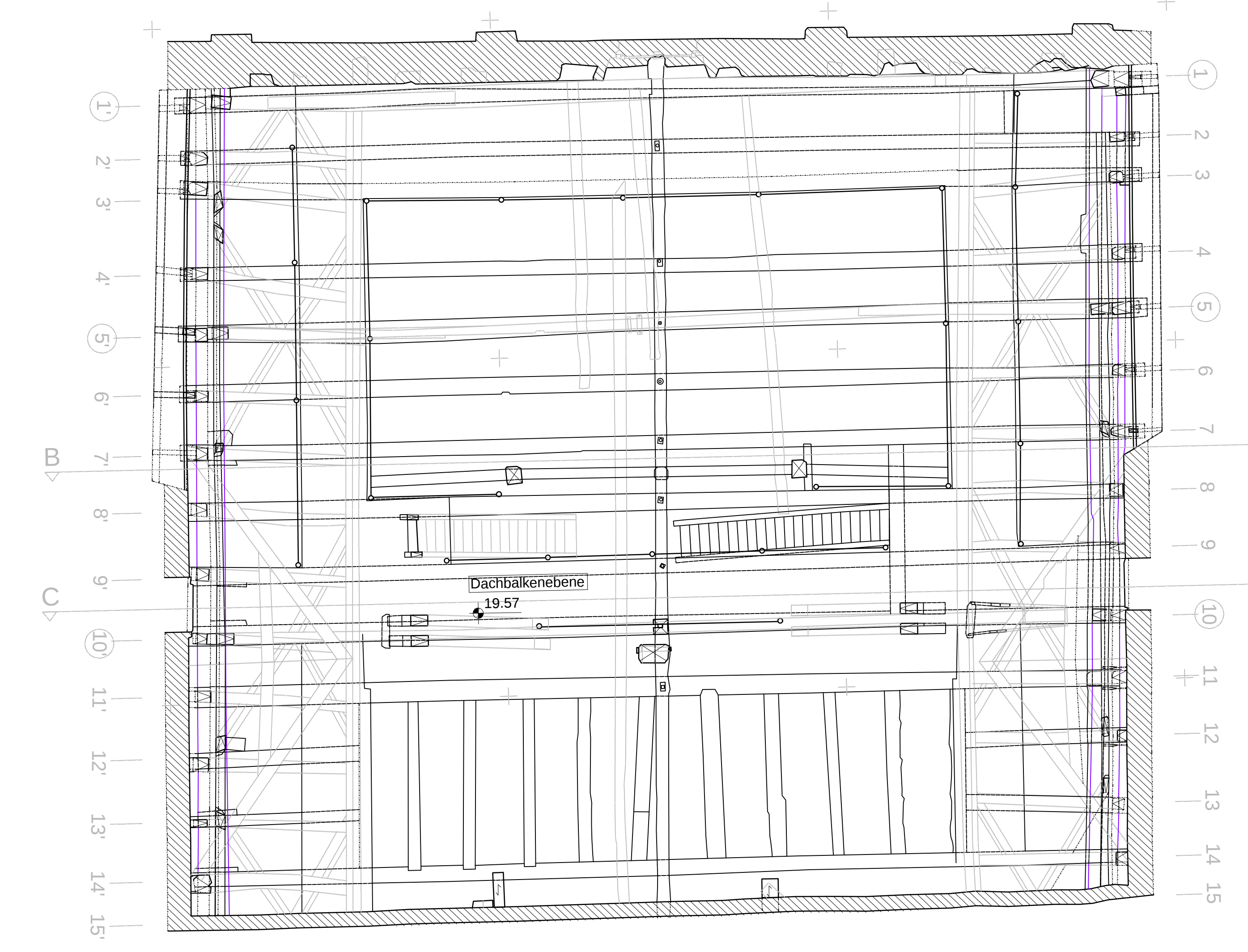
TREPPENHAUS GRUNDRISS DACHBALKENEbene DABE M 1:50
