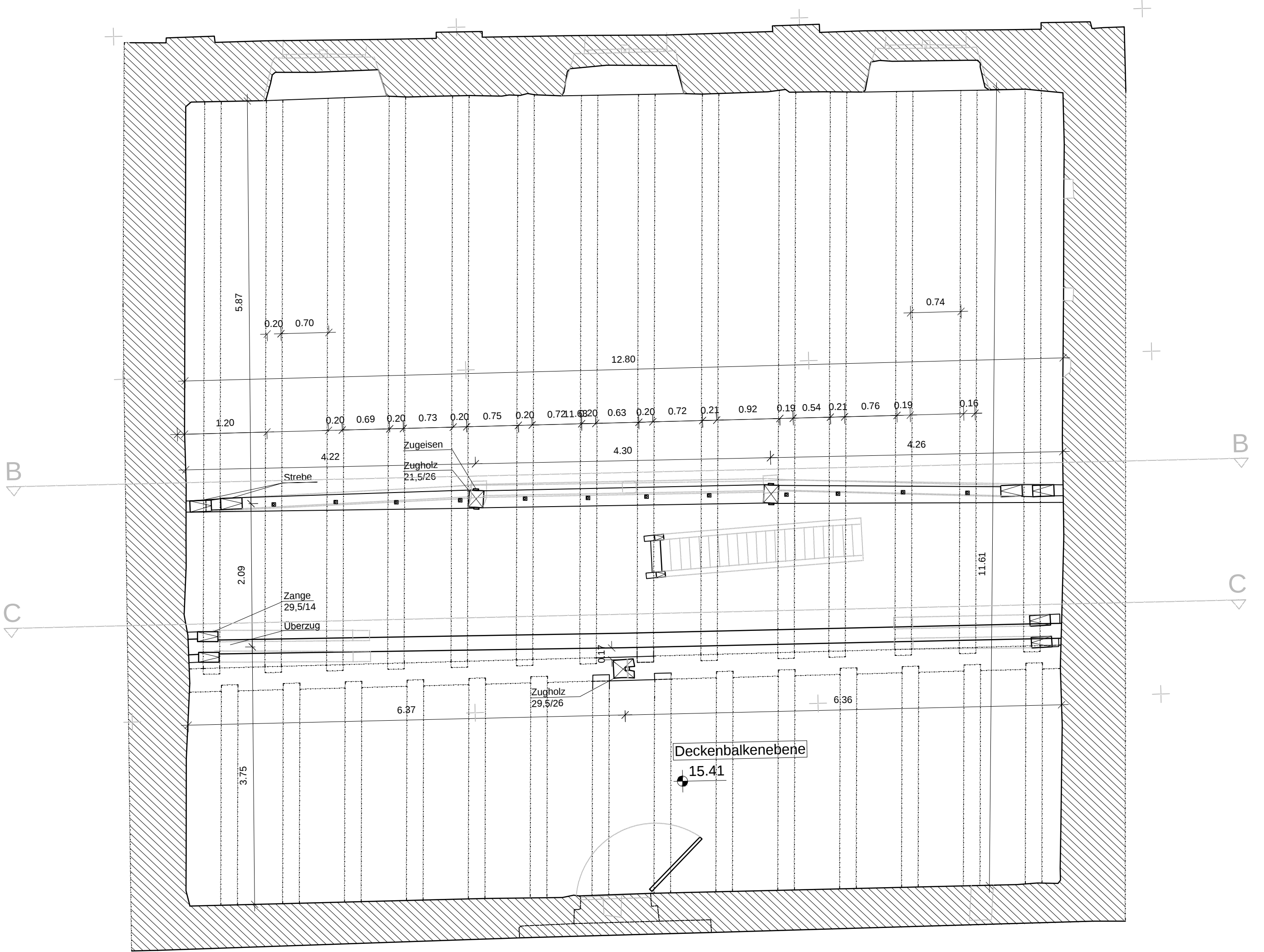
TREPPENHAUS GRUNDRISS DECKENBALKENEbene DEBE M 1:50
