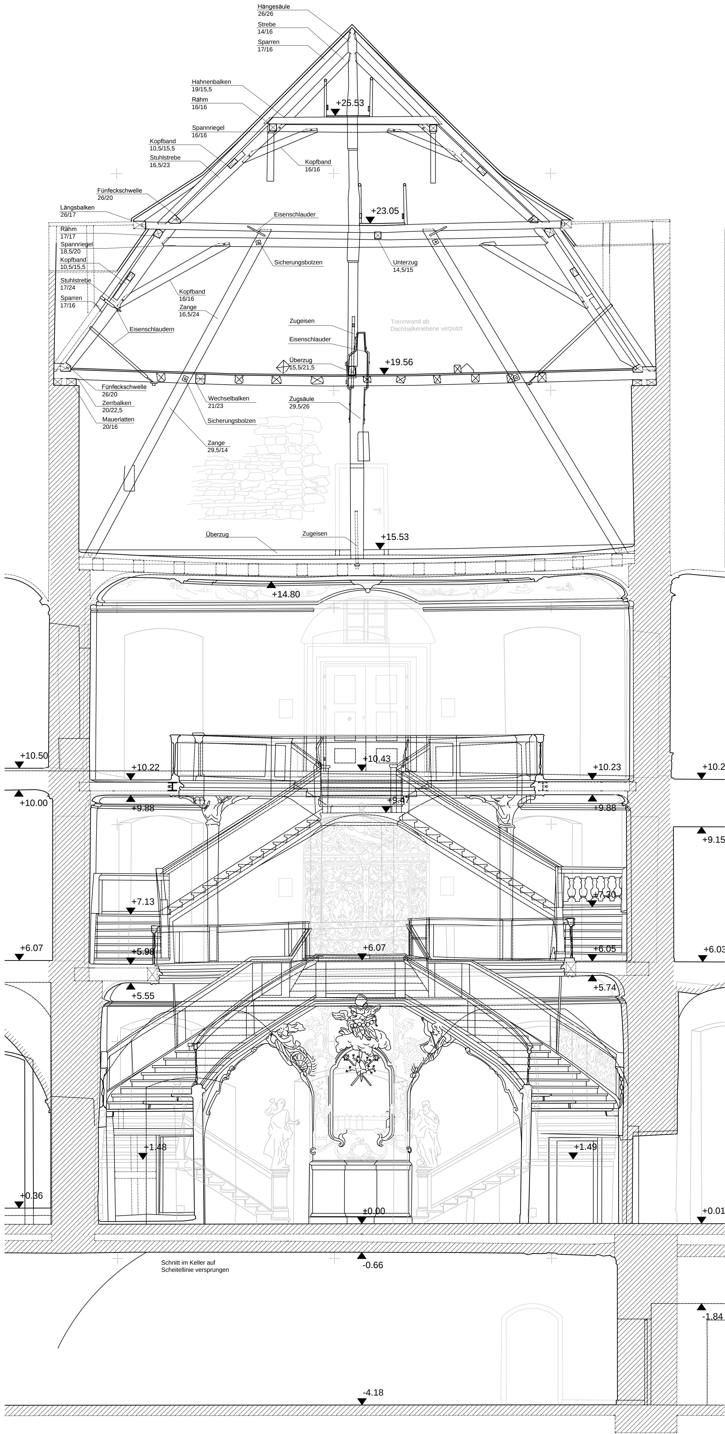
TREPPENHAUS SCHNITT A-A DACHSTUHL SCHNITT B-B M 1:50
