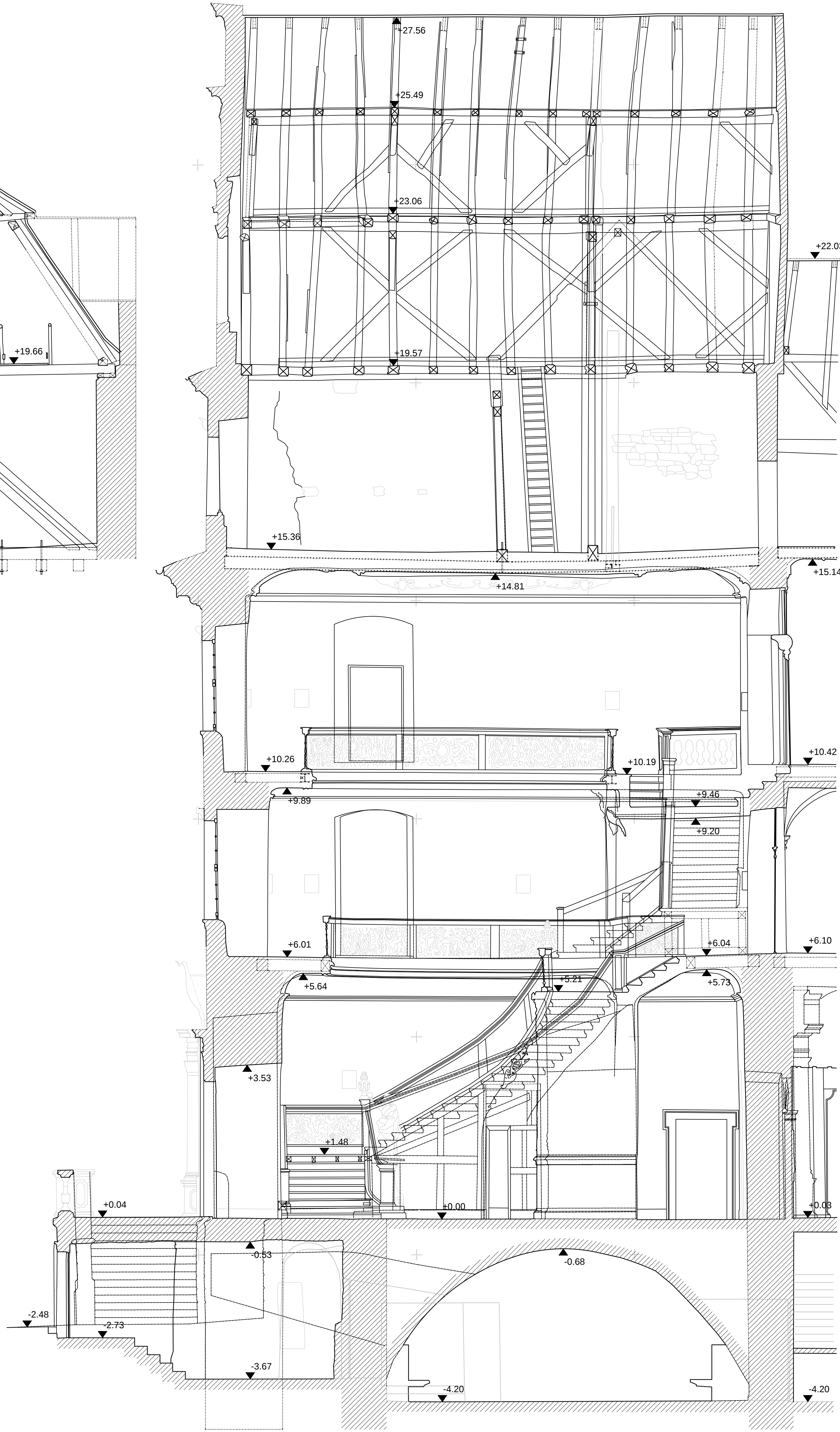
TREPPENHAUS SCHNITT D-D M 1:50
