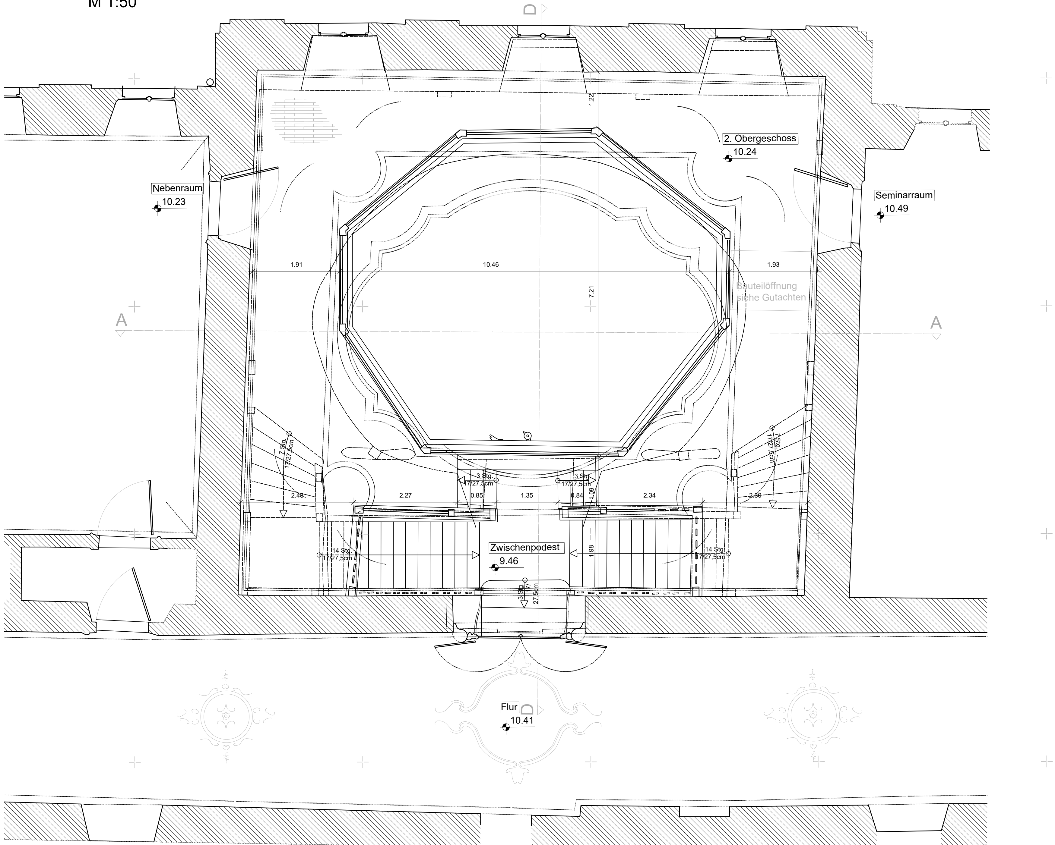
TREPPENHAUS GRUNDRISS 2. OBERGESCHOSS M 1:50
